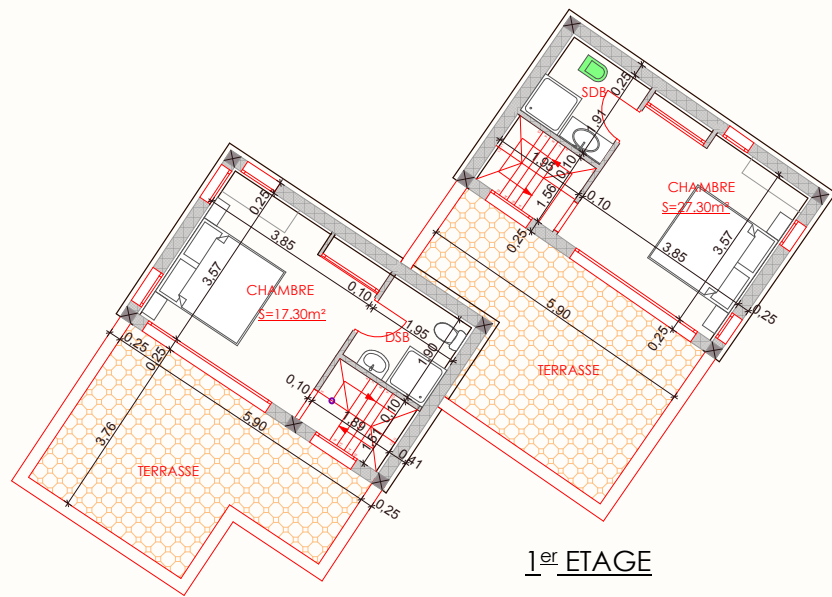
1 er Etage
